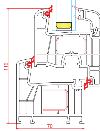
► 70 mm Çerçeve Kanat Montajı
