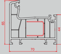
► Kanat Profili / 5 Odacık
