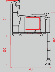
► Eşikli Çerçeve Profili
