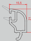
► 24 mm İkili Cam Çıtası
