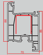
► Kapı Kanat Profili / 3 Odacık
