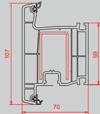
► Dışa Açılan Kapı Kanat Profili
