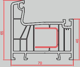
► Çerçeve Profili / 6 Odacık
