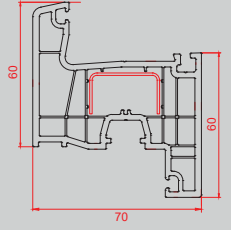
► Kanat Profili
