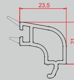
► 32 mm Üçlü Cam Çıtası
