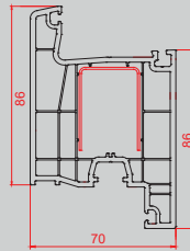
► Kapı Kanat Profili / 4 Odacık
