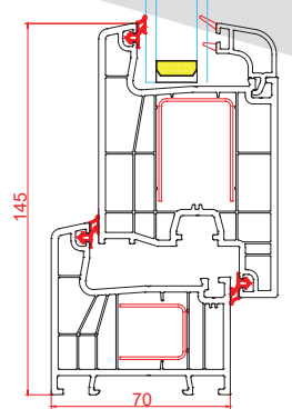
► 70 mm Çerçeve Kapı Kanat Montajı
