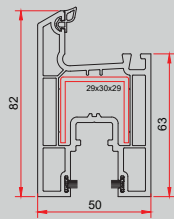
► Kayar Sistem Sash Profili
