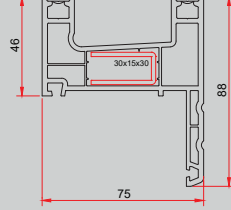
► Eşikli Çerçeve Profili (Dekoratif)
