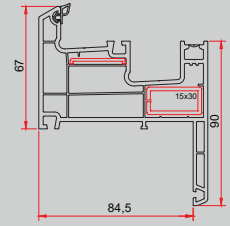
► Eşikli Çerçeve Profili (Tek Ray)
