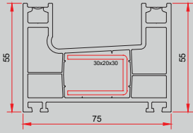
► Çerçeve Profili / Çift Ray
