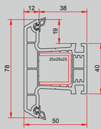
► 322 Sütun Profili
