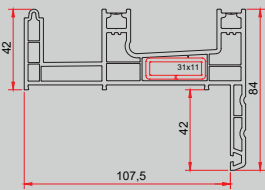
► Sinek Perdesi Eşikli Çift Raylı Çerçeve Profili (60 mm Eşik)
