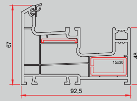
► Çerçeve Profili / Tek Ray
