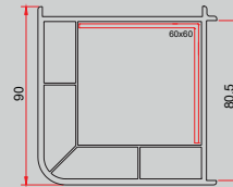
► 90° Köşe Profili
