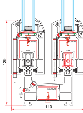
► Kayar Çerçeve Kanat Çift Ray Montajı
