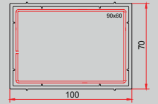
► Kutu Profili
